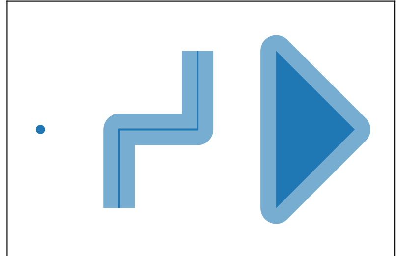
s.buffer(0.2, cap_style="flat")
